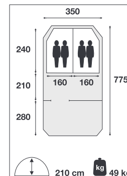
Baco optionele koppelkit
