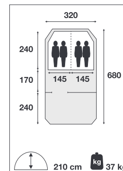
De ingang is eenvoudig drempelvrij te maken
